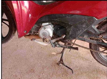
PANORAMICA MOTOR ESQUERDA
