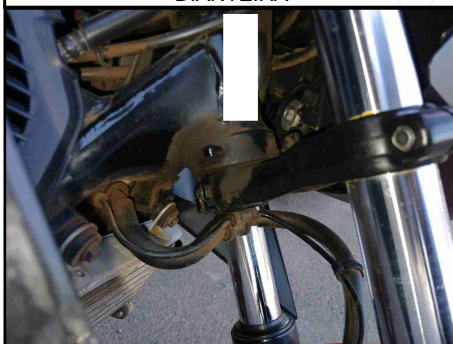
MESA INFERIOR DA SUSPENSÃO DIANTEIRA
