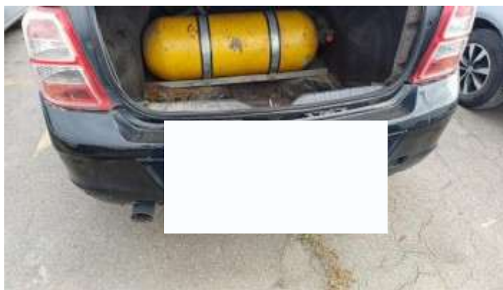
Para-choque traseiro
