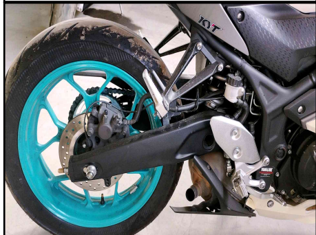
GARFO/BALANÇA TRASEIRO LADO DIREITO
