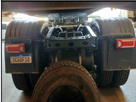
PARACHOQUE TRASEIRO
