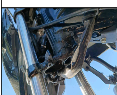
MESA INFERIOR SUSPENSÃO DIANTEIRA
