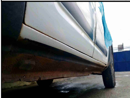
CAIXA DE AR/SOLEIRA DIREITA
