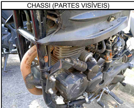
CHASSI (PARTES VISÍVEIS)
